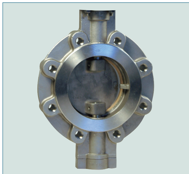
Konstrukce s děleným hřídelem nabízí lepší hodnoty průtoku při provozních tlacích do max. 19 bar.
